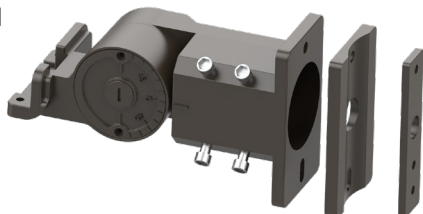
Ensemble pour têtes multiples
